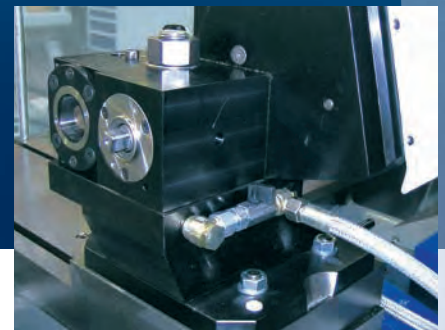
Werkzeugträgerkopf zum Drehen, Bohren und Fräsen
