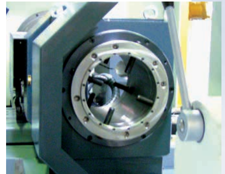
Ringlünette mit 270 mm Durchmesser
