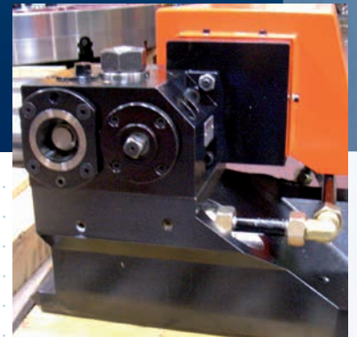
Werkzeugträgerkopf mit angetriebenen Werkzeugen, Aufnahme Capto C8
