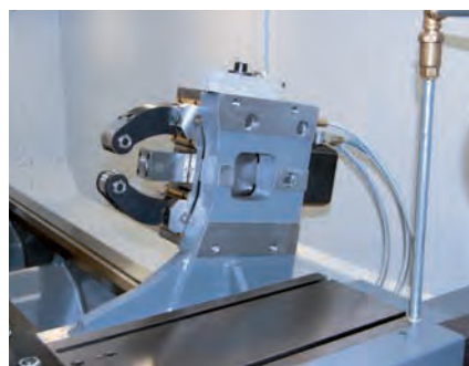
Mitlaufende, selbstzentrierende Lünette, hydraulisch betätigt
