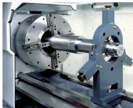
Pneumatisch betätigtes Vorderendfutter und feststehende Lünette
