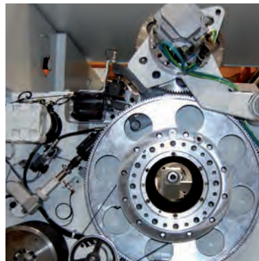
Einschwenkbare C-Achse
